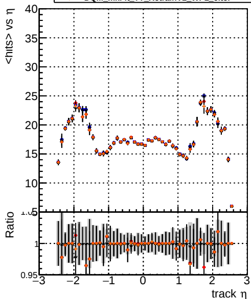
mean hits DQM_mkFit_TTbase DQM_mkFit_TT_retrainOldFiles125_v2_prelimWP_5iter DQM_mkFit_TT_baseline_6iter DQM_mkFit_TT_RetrainV2_WP2_6iter
