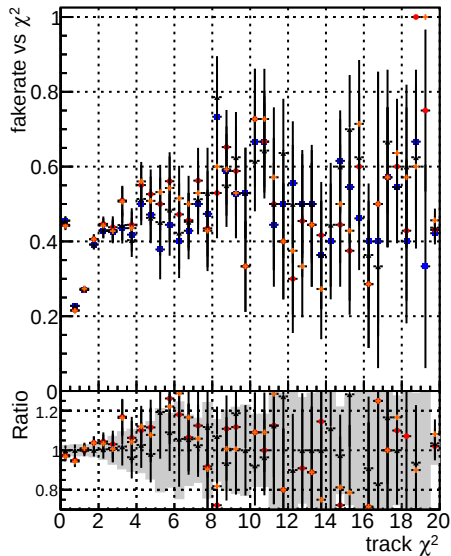
Fake rate vs. DGM mkFit Ttbase RetrainOldFiles125 v2 prelimWP_5iter DGM mkFit RetrainV2 WP2 6iter
