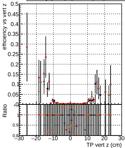
Efficiency vs vert z DOM_mkFit TTbase DOM_mkFit TT_retrainOldFiles125_v2_prelimWP_5iter DOM_mkFit TT_baseline_6iter DOM_mkFit TT_RetrainV2_WP2_6iter
