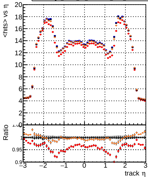
mean hit DQM_mkFit_TTbase DQM_mkFit_TT_retrainOldFiles125_v2_prelimWP_5iter DQM_mkFit_TT_baseline_6iter DQM_mkFit_TT_RetrainV2_WP2_6iter
