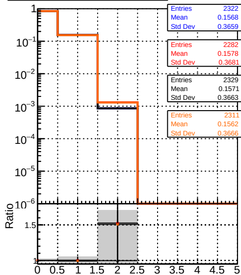
mean hits DQM_mkFit_TTbase DQM_mkFit_TT_retrainOldFiles125_v2_prelimWP_5iter DQM_mkFit_TT_baseline_6iter DQM_mkFit_TT_RetrainV2_WP2_6iter
