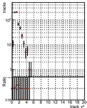
N of reco track vs. \chi^2 BGM mFit \chi^2 base BGM mFit \chi^2 base + 125 v2 prelinWP_5iter BGM mFit \chi^2 base + 125 v2 prelinWP_5iter + Retrain v2 WP2 6iter
