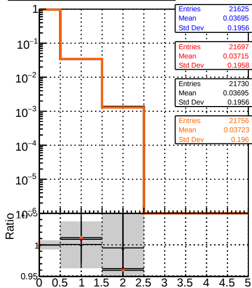
mean hit DQM_mkFit_TTbase DQM_mkFit_TT_retrainOldFiles125_v2_prelimWP_5iter DQM_mkFit_TT_baseline_6iter DQM_mkFit_TT_RetrainV2_WP2_6iter
