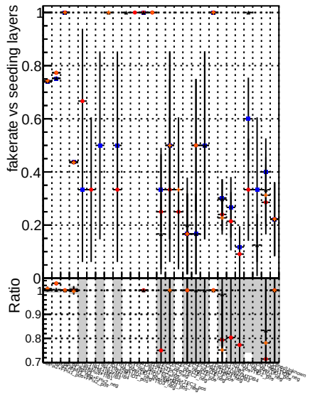
Fake rate vs. BGM mkFit TTbase BGM mkFit RetrainOldFiles125 v2 prelimWP_5iter BGM mkFit RetrainV2 WP2 6iter
