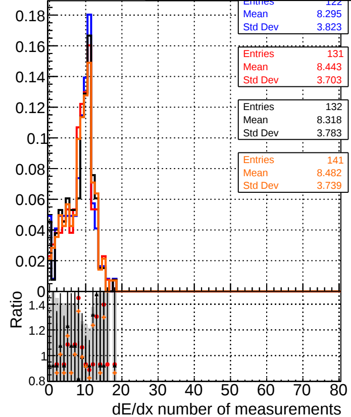
—■— DQM_mkFit_TTbase —●— DQM_mkFit_TT_retrainOldFiles125_v2_prelimWP_5iter —▲— DQM_mkFit_TT_baseline_6iter —◆— DQM_mkFit_TT_RetrainV2_WP2_6iter
