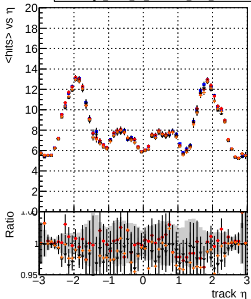
mean hits vs \eta DQM_mkFit_TTbase DQM_mkFit_TT_retrainOldFiles125_v2_prelimWP_5iter DQM_mkFit_TT_baseline_6iter DQM_mkFit_TT_RetrainV2_WP2_6iter
