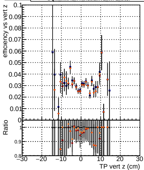
Efficiency vs vert z —●— DQM_mkFit_TTbase —▲— DQM_mkFit_TT_retrainOldFiles125_v2_prelimWP_5iter —▼— DQM_mkFit_TT_baseline_6iter —◆— DQM_mkFit_TT_RetrainV2_WP2_6iter
