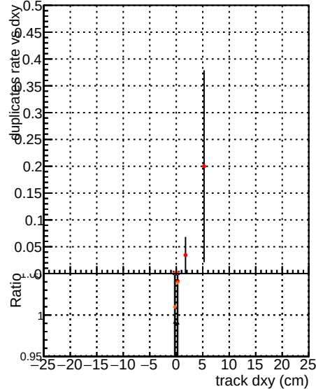
Legend: DQM mktFit Tbase Data OldFiles125 v2 prelimWP_5iter DQM mktFit RetrainV2 WP2_6iter
