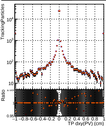
— DQM_mkFit_TTbase — DQM_mkFit_TT_retrainOldFiles125_v2_prelimWP_5iter — DQM_mkFit_TT_baseline_6iter — DQM_mkFit_TT_RetrainV2_WP2_6iter
