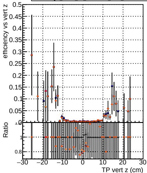
Efficiency vs. TP vert z (cm) DOM_mkFit TTbase DOM_mkFit TT_retrainOldFiles125_v2_prelimWP_5iter DOM_mkFit TT_baseline_6iter DOM_mkFit TT_RetrainV2_WP2_6iter
