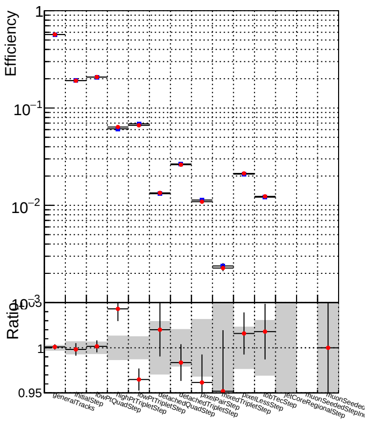
DQM_mkFit_TTbase DQM_mkFit_TT_retrainOldFiles125_v2_prelimWP_5iter
