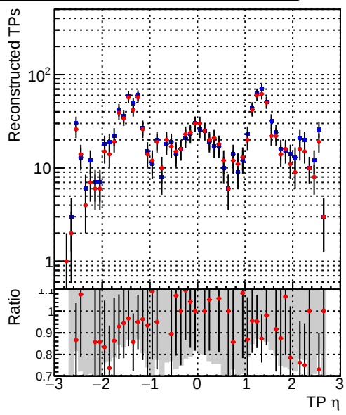
Legend: — DQM_mkFit_TTbase — DQM_mkFit_TT_retrainOldFiles125_v2_prelimWP_5iter
