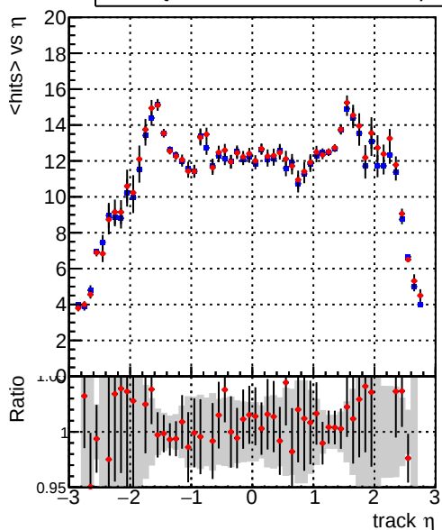
mean hit — DQM_mkFit_TTbase — DQM_mkFit_TT_retrainOldFiles125_v2_prelimWP_5iter
