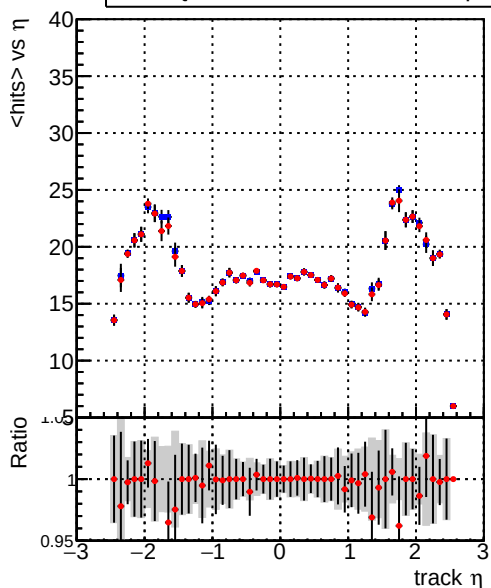
mean hits — DQM_mkFit_TTbase — DQM_mkFit_TT_retrainOldFiles125_v2_prelimWP_5iter
