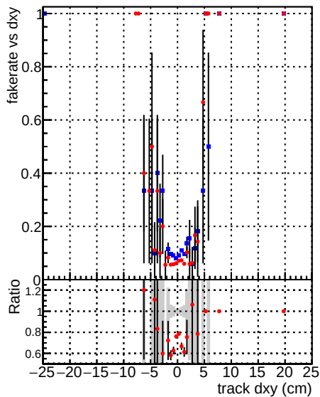
—●— DQM_mkFit_TTbase —●— DQM_mkFit_TT_retrainOldFiles125_v2_prelimWP_5iter
