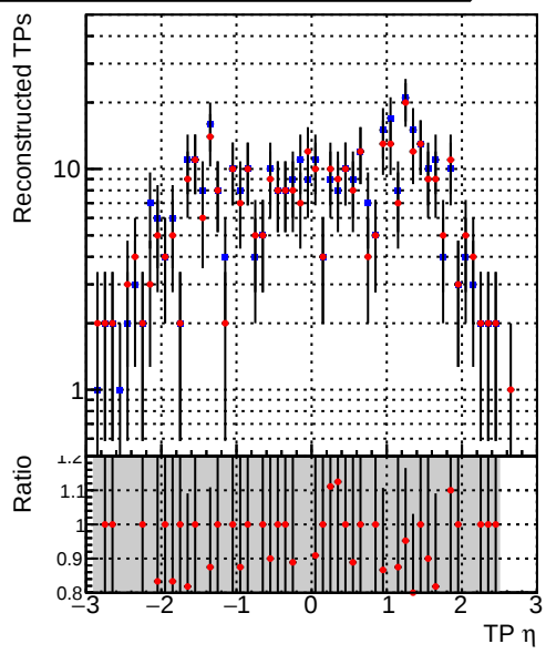
—•— DQM_mkFit_TTbase —•— DQM_mkFit_TT_retrainOldFiles125_v2_prelimWP_5iter
