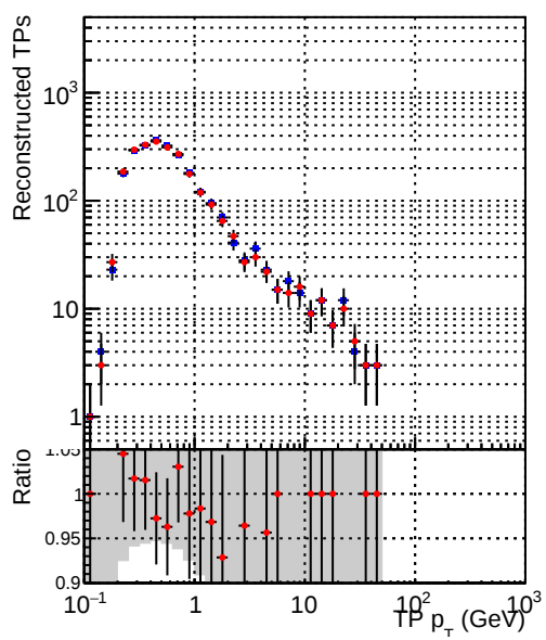
—•— DQM_mkFit_TTbase —•— DQM_mkFit_TT_retrainOldFiles125_v2_prelimWP_5iter
