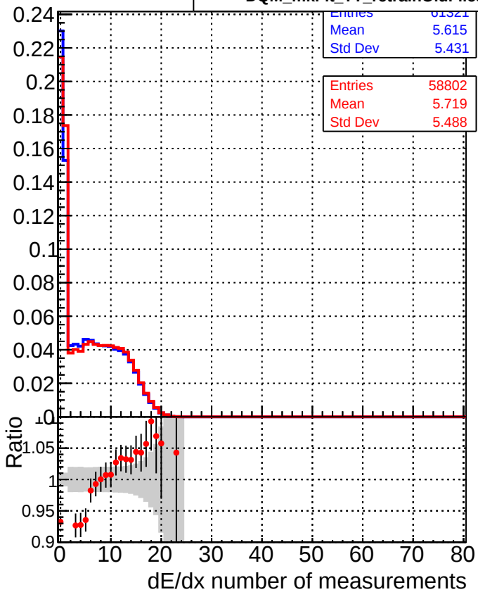
■ DQM_mkFit_TTbase ● DQM_mkFit_TT_retrainOldFiles125_v2_prelimWP_5iter
