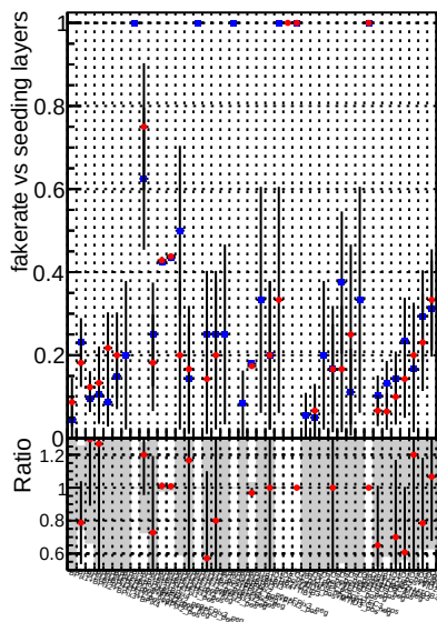
Fake rate vs. —♦— DQM mkFit TTbase —★— DQM mkFit TT_retrainOldFiles125_v2_prelimWP_5iter
