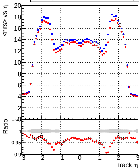
— DQM_mkFit_TTbase — DQM_mkFit_TT_retrainOldFiles125_v2_prelimWP_5iter
