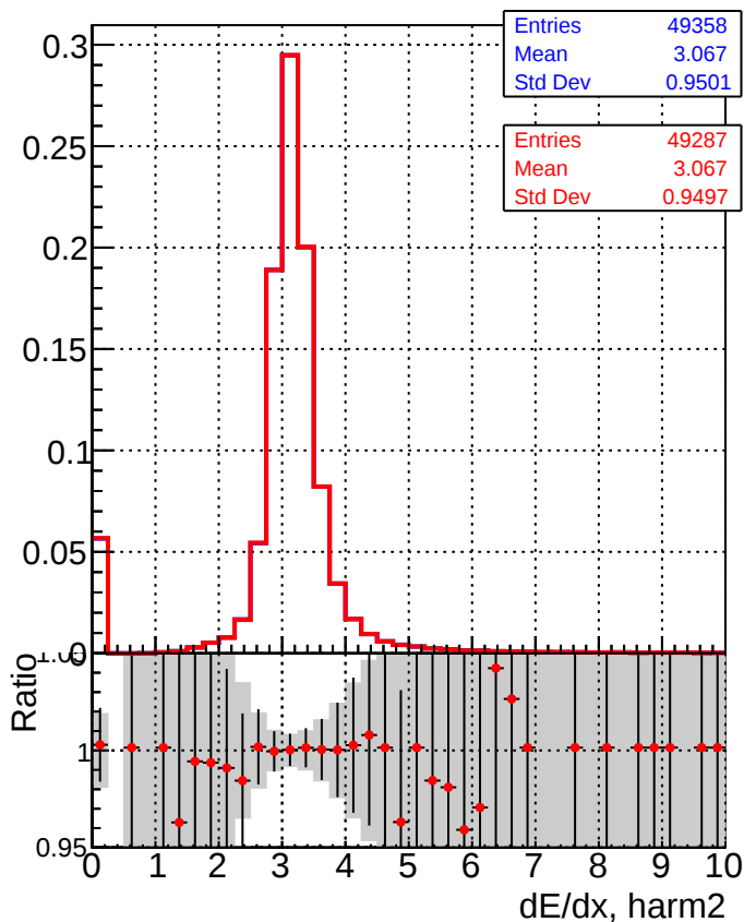
■ DQM_mkFit_TTbase —●— DQM_mkFit_TT_retrainOldFiles125_v2_prelimWP_5iter
