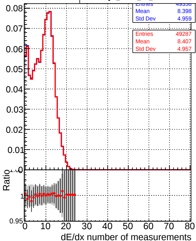
■ DQM_mkFit_TTbase —●— DQM_mkFit_TT_retrainOldFiles125_v2_prelimWP_5iter
