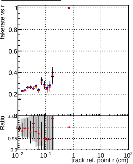
Fake rate vs v —●— DQM_mkFit_TTbase —●— DQM_mkFit_TT_retrainOldFiles125_v2_prelimWP_5iter
