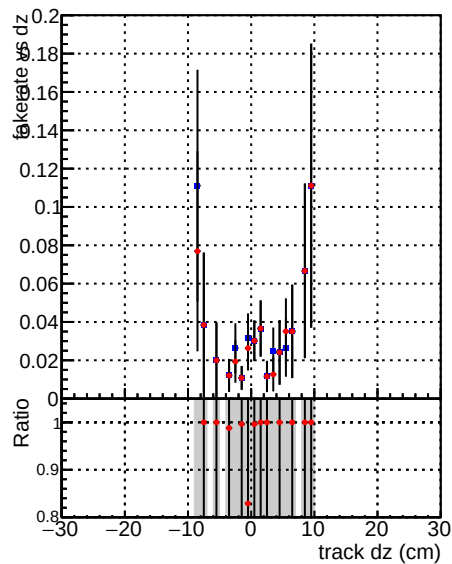
—•— DQM_mkFit_TTbase —•— DQM_mkFit_TT_retrainOldFiles125_v2_prelimWP_5iter
