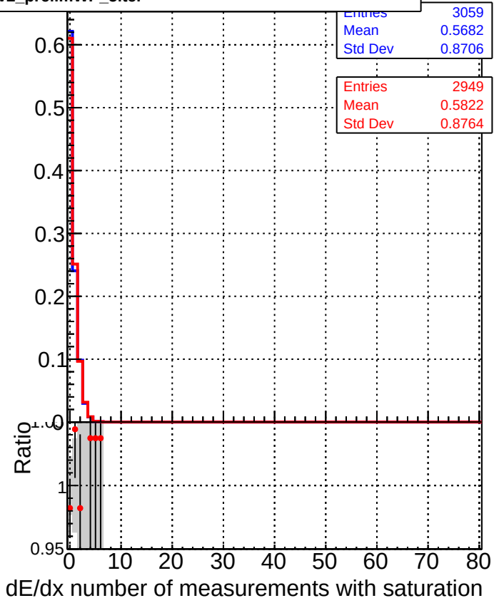
■ DQM_mkFit_TTbase ● DQM_mkFit_TT_retrainOldFiles125_v2_prelimWP_5iter
