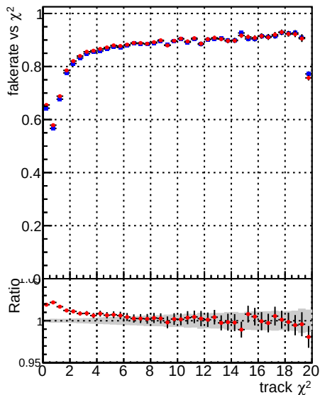
Fake rate vs. — DQM_mkFit_TTbase — DQM_mkFit_TT_retrainOldFiles125_v2_prelimWP_5iter
