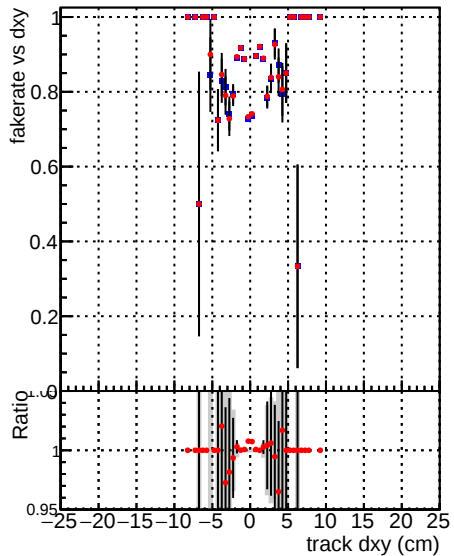
—●— DQM_mkFit_TTbase —●— DQM_mkFit_TT_retrainOldFiles125_v2_prelimWP_5iter
