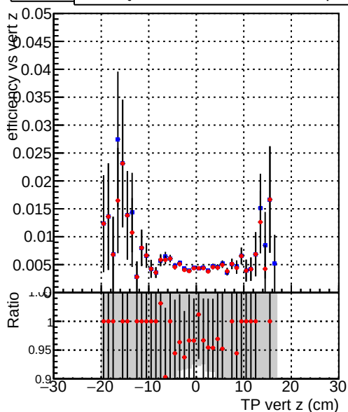
Efficiency vs vert z —●— DQM_mkFit_TTbase —●— DQM_mkFit_TT_retrainOldFiles125_v2_prelimWP_5iter
