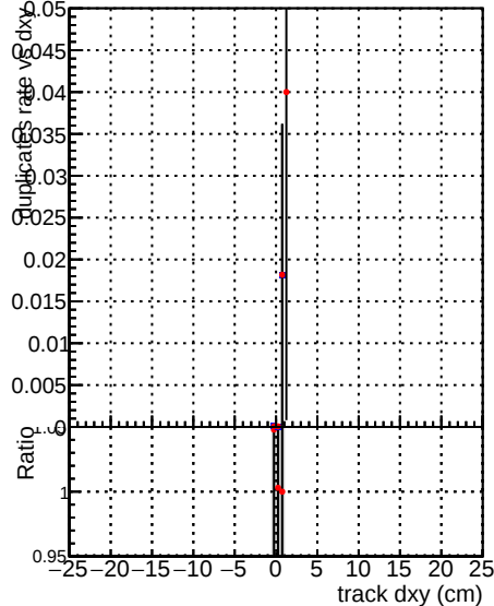
—●— DQM_mkFit_TTbase —●— DQM_mkFit_TT_retrainOldFiles125_v2_prelimWP_5iter
