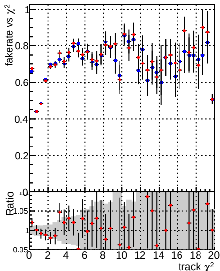
Fake rate vs. —◆— DQM mkFit TTbase —●— DQM mkFit TT_retrainOldFiles125_v2_prelimWP_5iter
