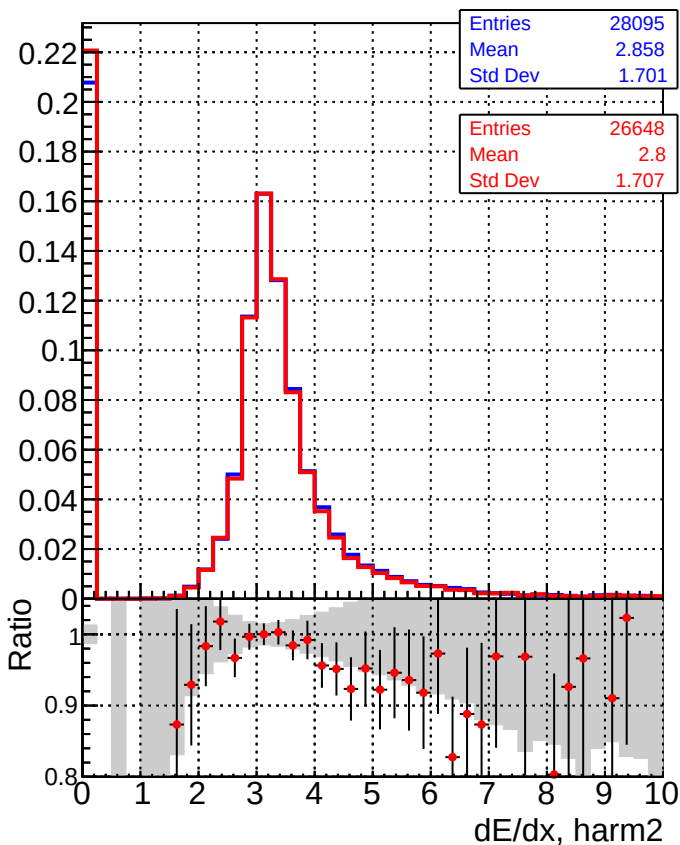
—■— DQM_mkFit_TTbase —●— DQM_mkFit_TT_retrainOldFiles125_v2_prelimWP_5iter
