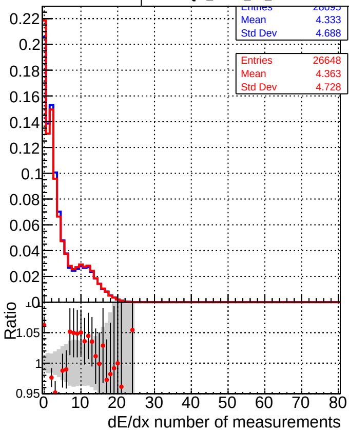
—■— DQM_mkFit_TTbase —●— DQM_mkFit_TT_retrainOldFiles125_v2_prelimWP_5iter
