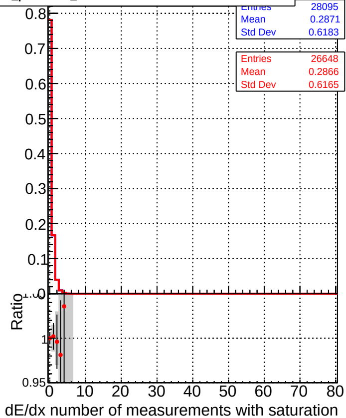
—■— DQM_mkFit_TTbase —●— DQM_mkFit_TT_retrainOldFiles125_v2_prelimWP_5iter
