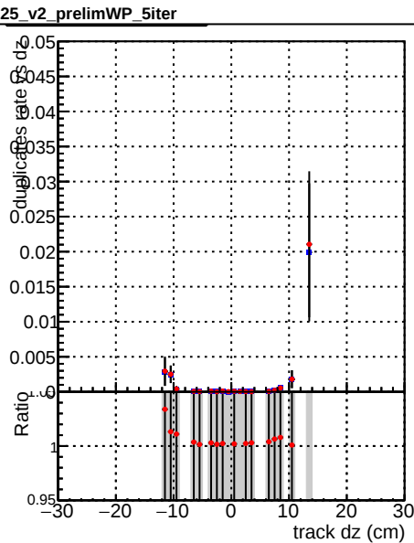
—●— DQM_mkFit_TTbase —●— DQM_mkFit_TT_retrainOldFiles125_v2_prelimWP_5iter
