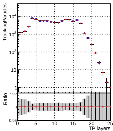
N of sim DQM_mkFit_TTbase DQM_mkFit_TT_retrainOldFiles125_v2_prelimWP_5iter
