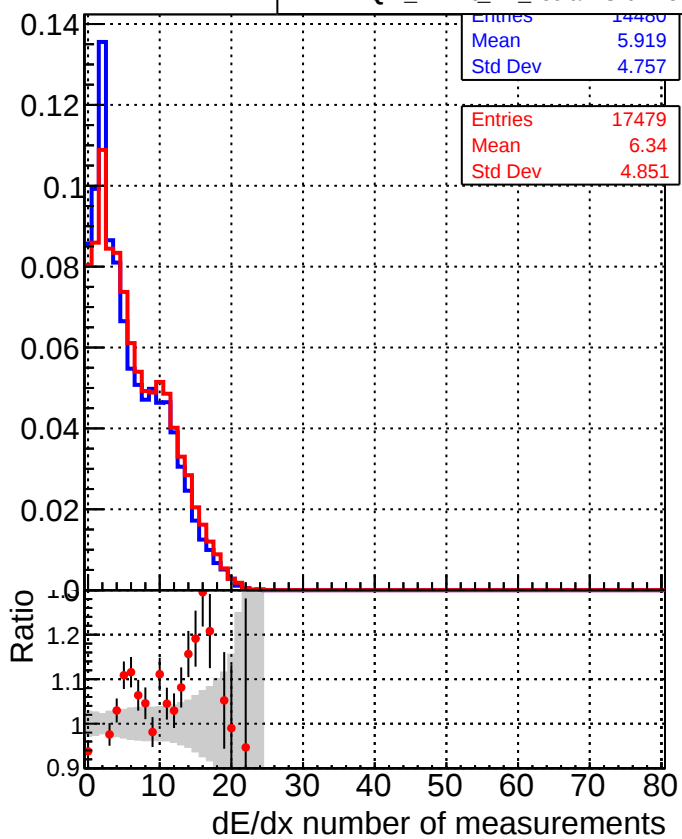
—■— DQM_mkFit_TTbase —●— DQM_mkFit_TT_retrainOldFiles125_v2_prelimWP_5iter
