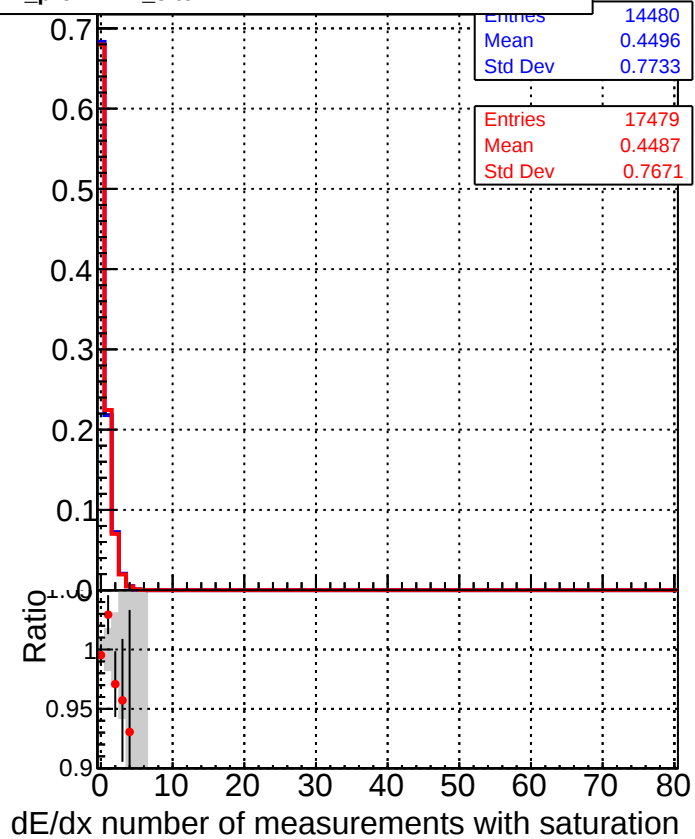
—■— DQM_mkFit_TTbase —●— DQM_mkFit_TT_retrainOldFiles125_v2_prelimWP_5iter
