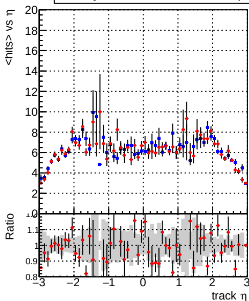
— DQM_mkFit_TTbase — DQM_mkFit_TT_retrainOldFiles125_v2_prelimWP_5iter mean hits
