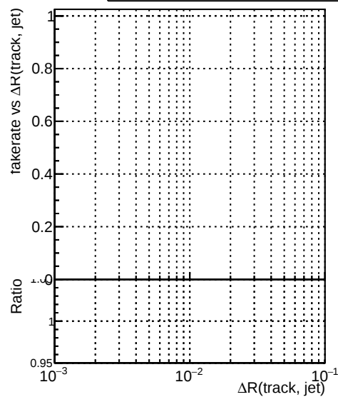
Legend: —•— DQM_mkFit_TTbase —•— DQM_mkFit_TT_retrainOldFiles125_v2_prelimWP_5iter
