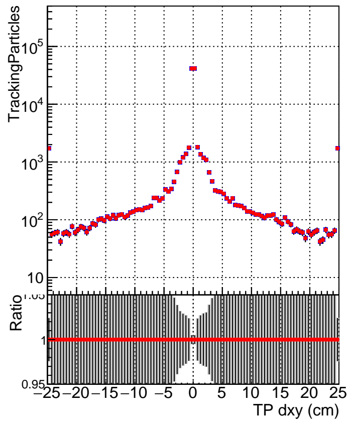
■ DQM_mkFit_TTbase ● DQM_mkFit_TT_retrainOldFiles125_v2_prelimWP
