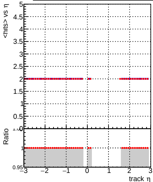
— DQM_mkFit_TTbase — DQM_mkFit_TT_retrainOldFiles125_v2_prelimWP
