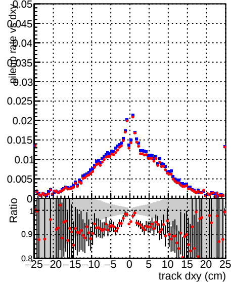
DQM_mkFit_TT_retrainOldFiles125_v2_prelimWP
