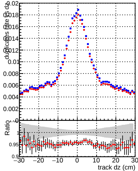
DQM_mkFit_TTbase
