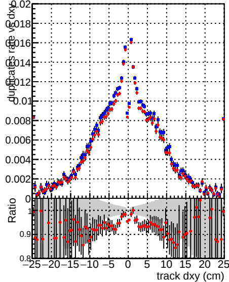
DQM_mkFit_TTbase
