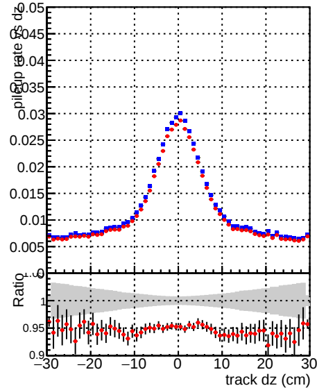
DQM_mkFit_TT_retrainOldFiles125_v2_prelimWP
