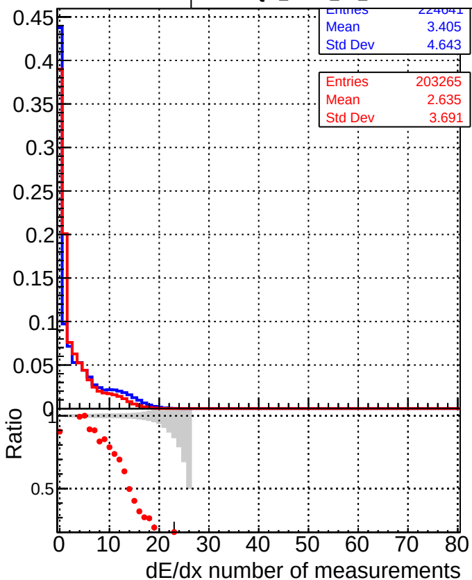
■ DQM_mkFit_TTbase ● DQM_mkFit_TT_retrainOldFiles125_v2_prelimWP
