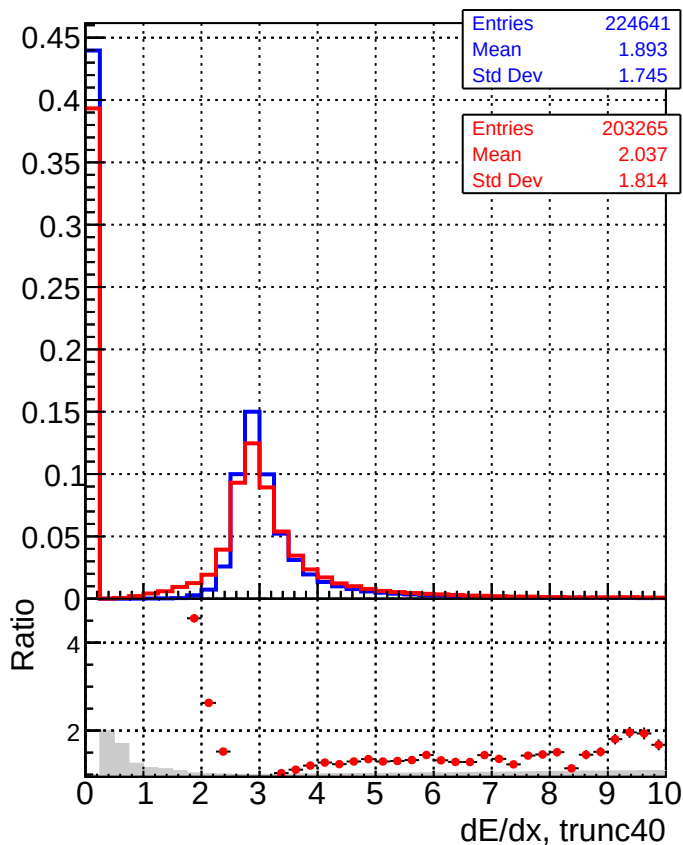
■ DQM_mkFit_TTbase ● DQM_mkFit_TT_retrainOldFiles125_v2_prelimWP
