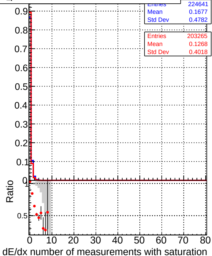
■ DQM_mkFit_TTbase ● DQM_mkFit_TT_retrainOldFiles125_v2_prelimWP
