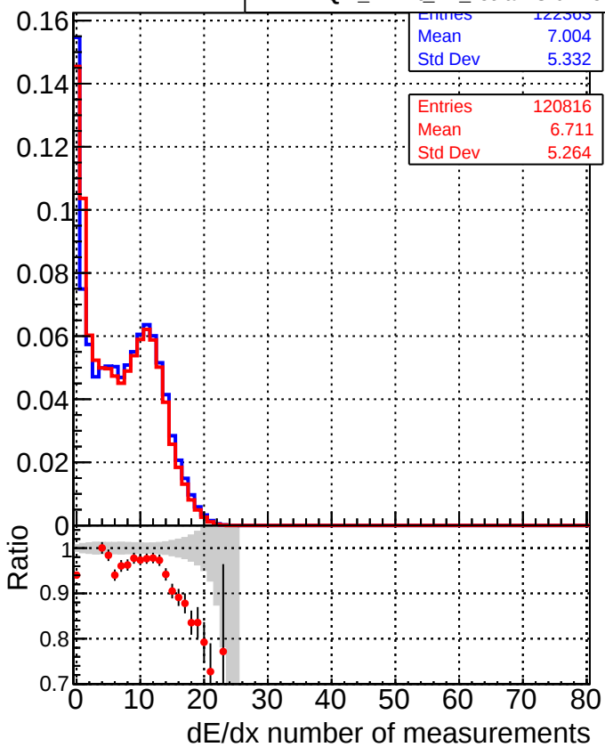
DQM_mkFit_TTbase DQM_mkFit_TT_retrainOldFiles125_v2_prelimWP
