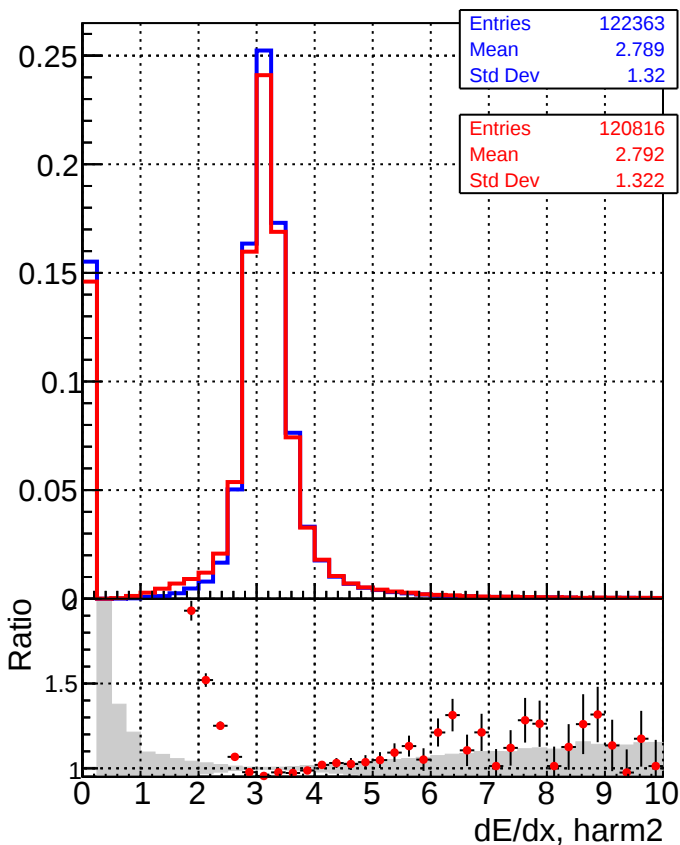
DQM_mkFit_TTbase DQM_mkFit_TT_retrainOldFiles125_v2_prelimWP
