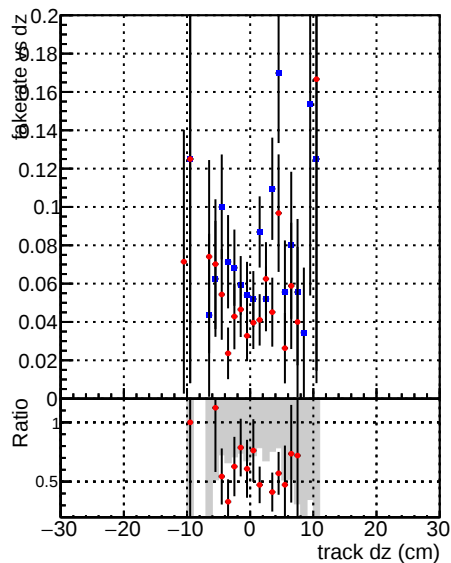
—●— DQM_mkFit_TTbase —●— DQM_mkFit_TT_retrainOldFiles125_v2_prelimWP
