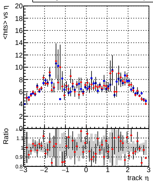
— DQM_mkFit_TTbase — DQM_mkFit_TT_retrainOldFiles125_v2_prelimWP
