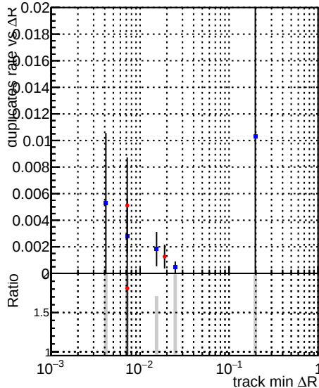
—●— DQM_mkFit_TTbase —●— DQM_mkFit_TT_retrainOldFiles125_v2_prelimWP
