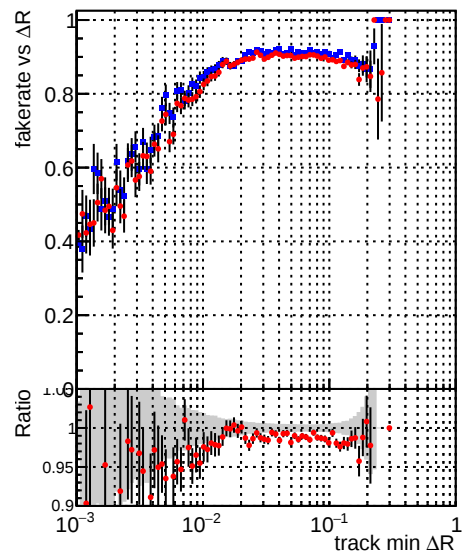
—●— DQM_mkFit_TTbase —●— DQM_mkFit_TT_retrainOldFiles125_v2_prelimWP
