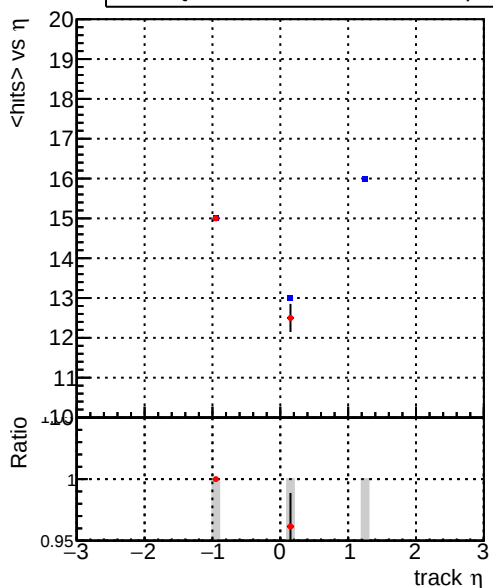
— DQM_mkFit_TTbase — DQM_mkFit_TT_retrainOldFiles125_v2_prelimWP
