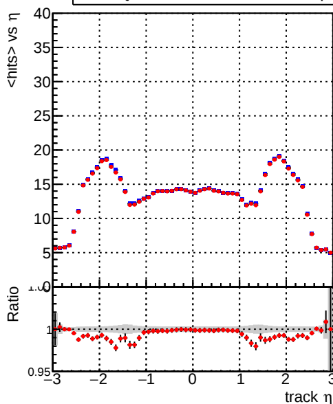
— DQM_mkFit_TTbase — DQM_mkFit_TT_retrainOldFiles125_v2_prelimWP
