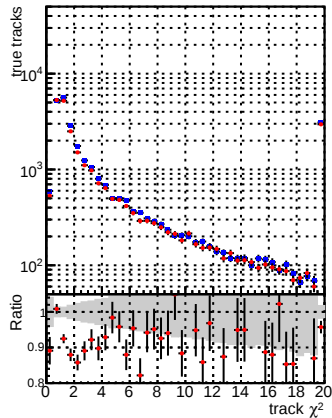
N of reco track vs. \chi^2 DQM mkFit TTbase DQM mkFit TT_retrainOldFiles125_v2_prelimWP
