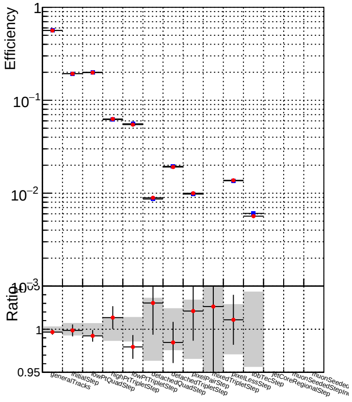
DQM_CKF_TTbase DQM_CKF_TT_retrainOldFiles125_v2_prelimWP_epoch4
